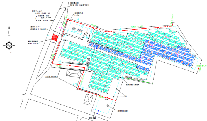
パネル配置
