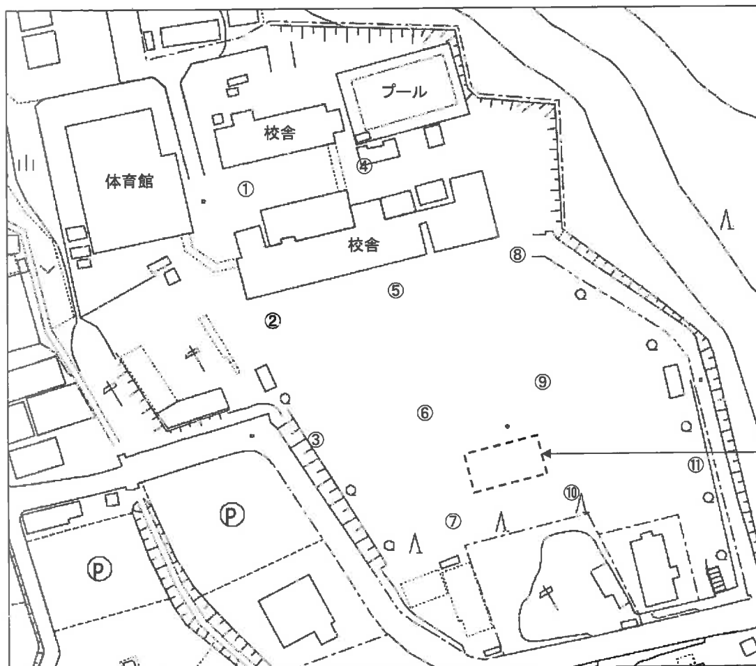
除染後放射線量マップ【酒井根西小学校】
