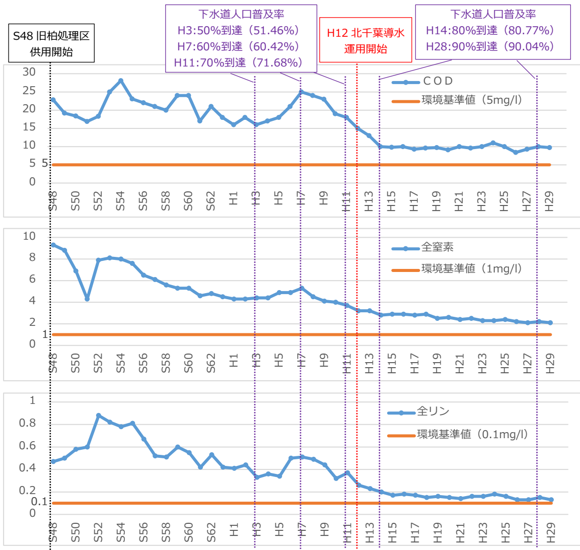
図 1-2-3-3 手賀沼中央の水質汚濁 (単位: mg/l) (出典: 柏市環境白書)
