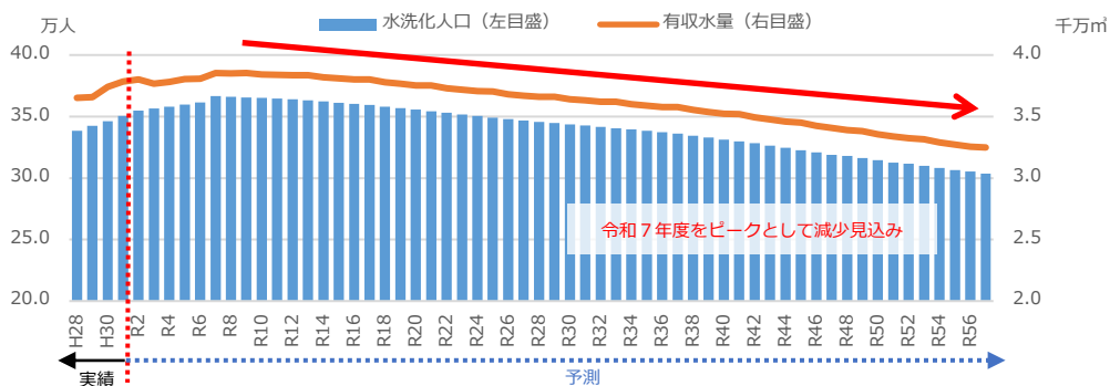
図 3-1-6-1 水化人口と有収水量の見通し
