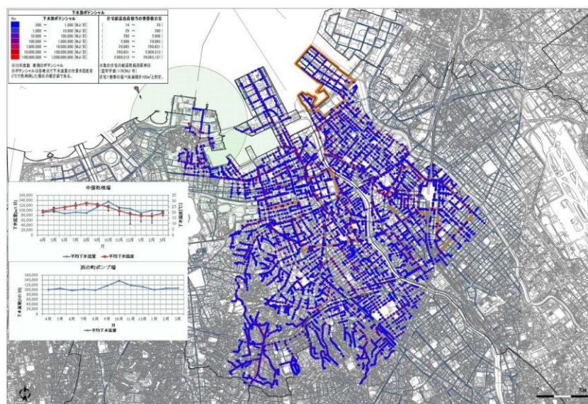
図 2-1-2-2 広域ポテンシャルマップの事例 出典：「下水熱ポテンシャルマップ（広域ポテンシャルマップ）作成の手引き」 （環境省総合環境政策局，国土交通省下水道部，2015）
