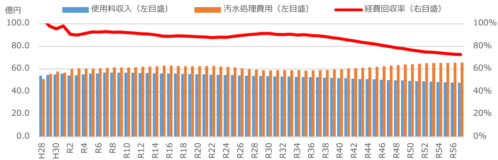
図 3-1-6-5 経費回収率の見通し
