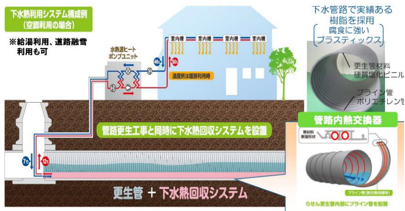
図 2-1-2-1 管路内設置型熱回収技術
