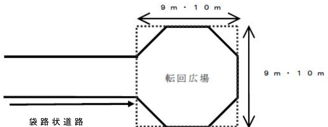
図 3 終端の転回広場 (ラウンド型)
