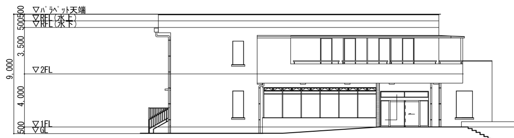
北側立面図
