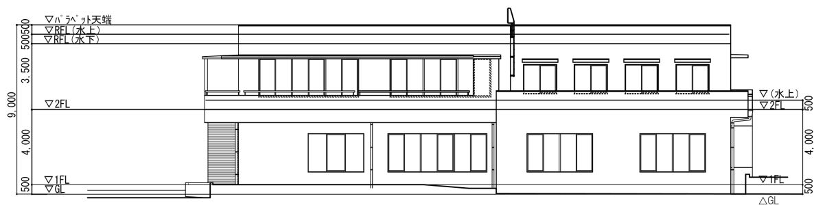
西側立面図
