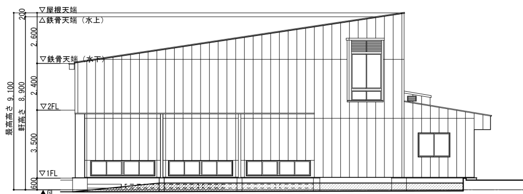
北側立面図
