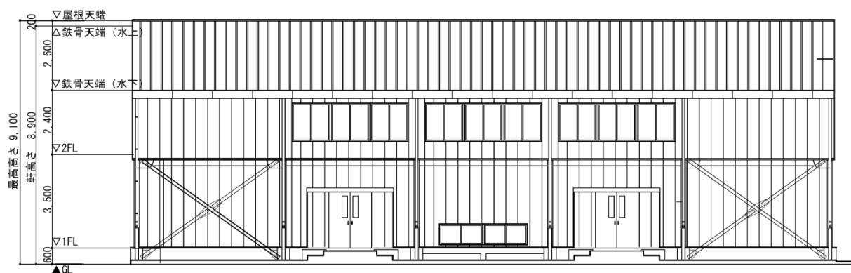
東側立面図
