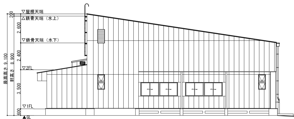
南側立面図
