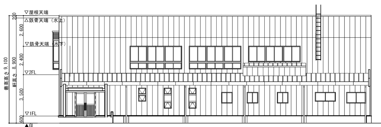
西側立面図
