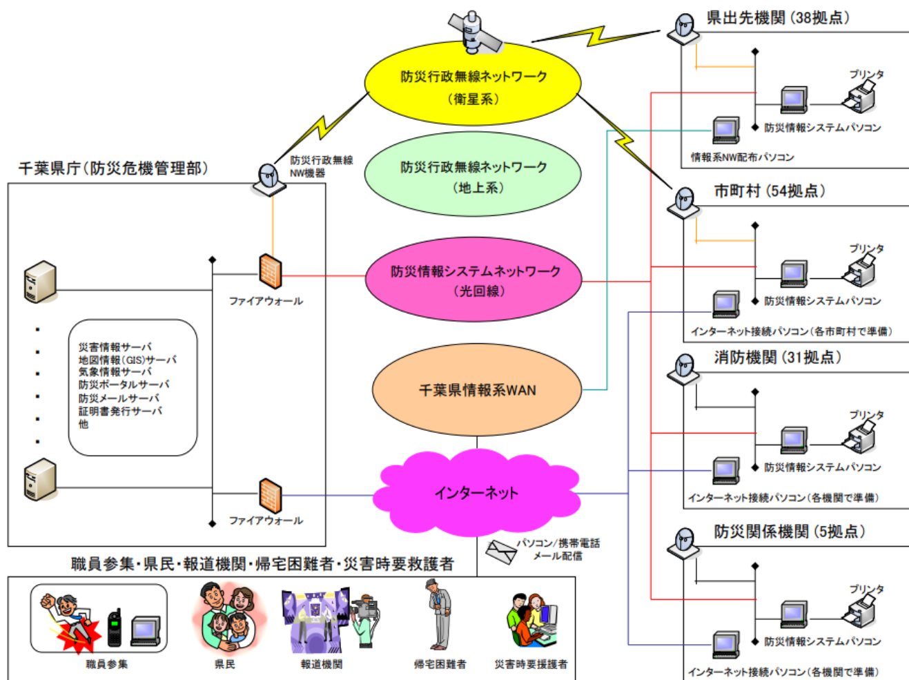
千葉県防災情報システム構成概念図（引用元：「千葉県地域防災計画資料編」）
