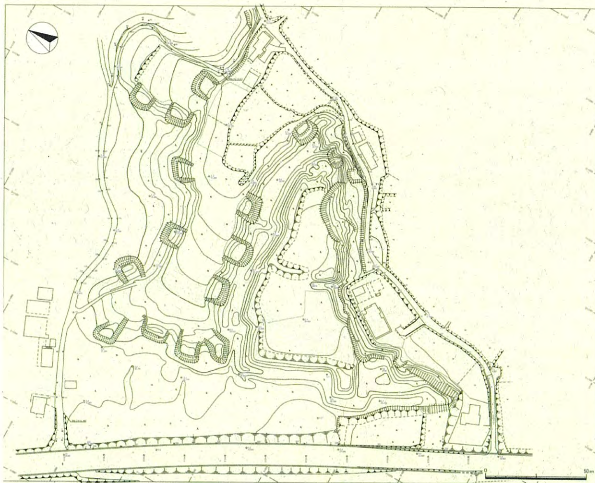
図2 増尾城跡実測図
