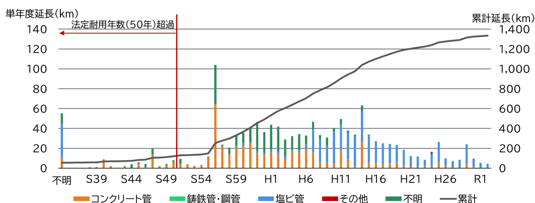
管路の布設年度別整備延長(上段:水道管路、下段:下水道管きょ)
