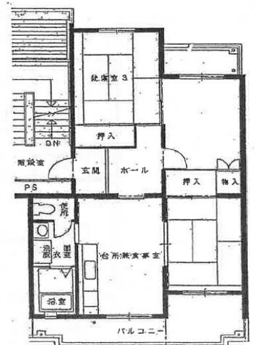
36 塚崎団地 1号棟 (3DK一般)
