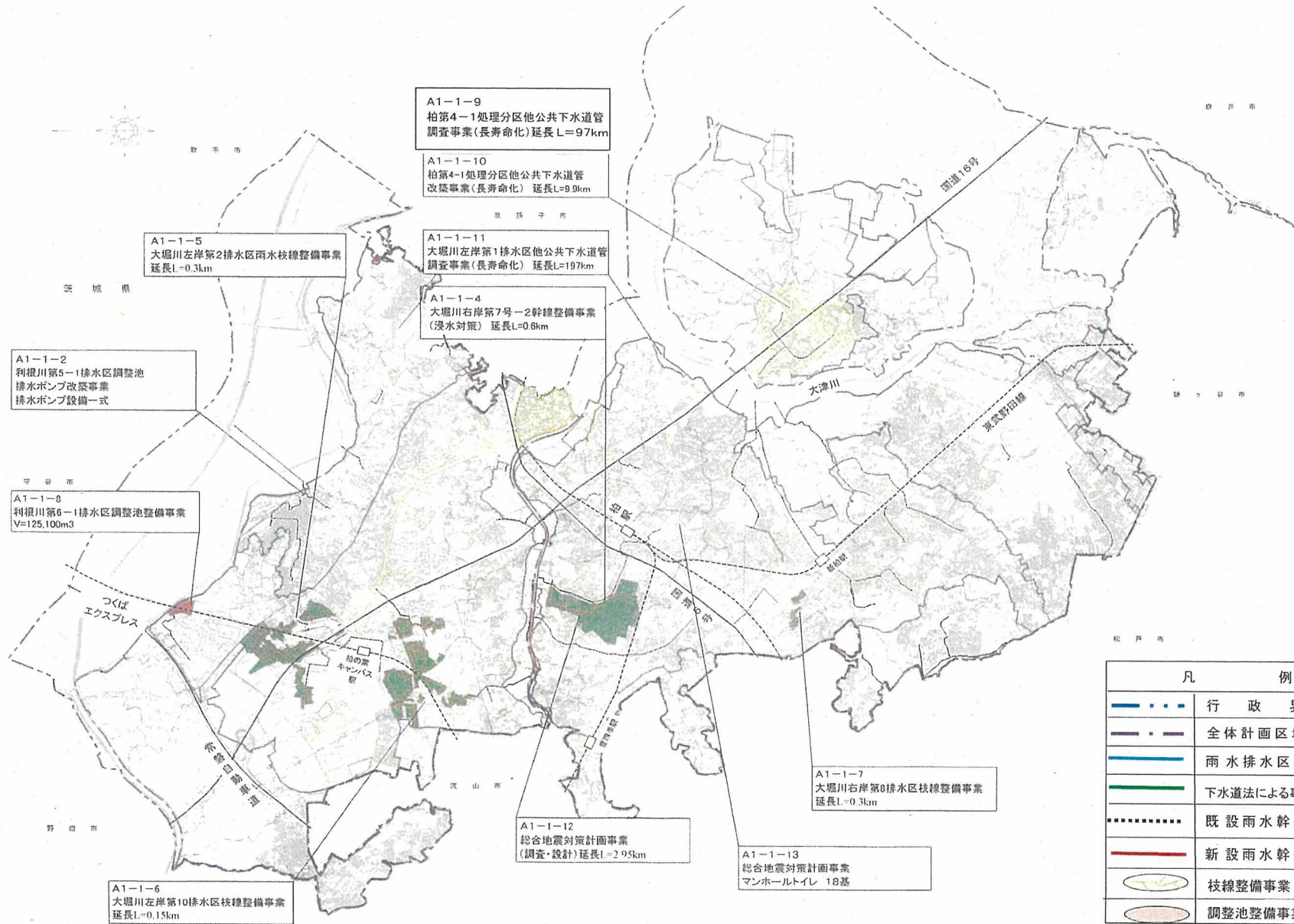
雨水排水計画図
