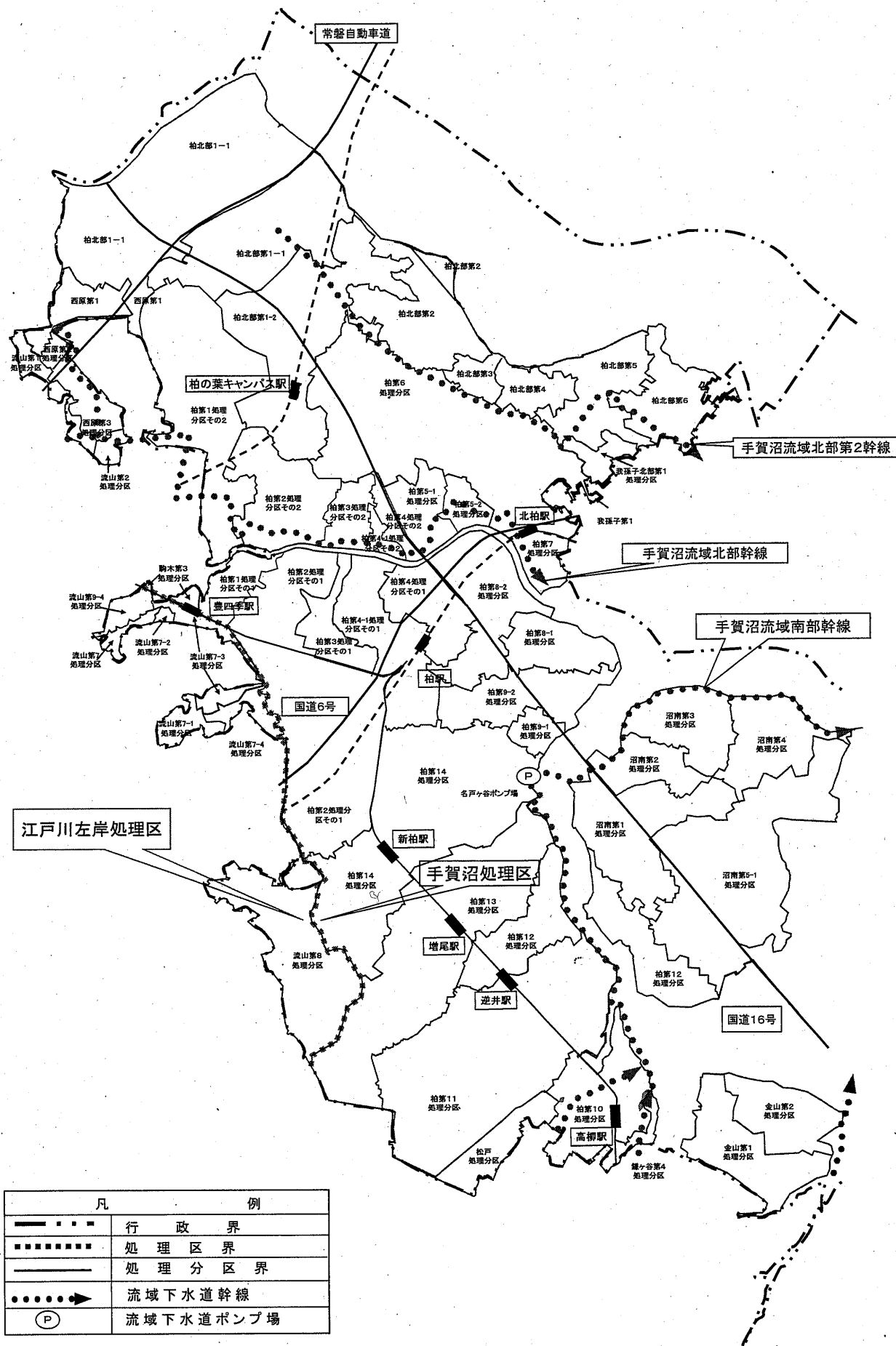
図1-1 汚水計画図
