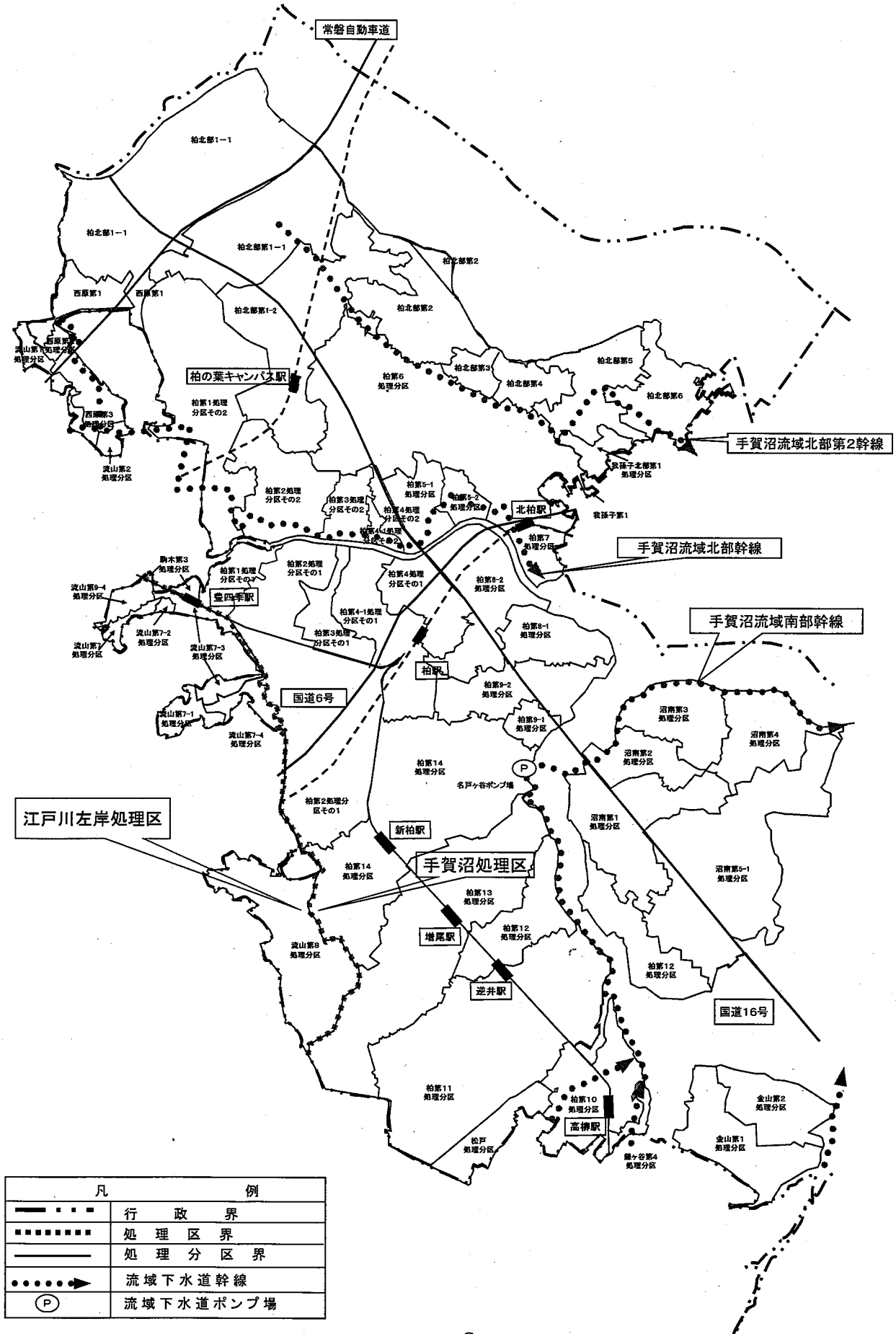
図1-1 汚水計画図
