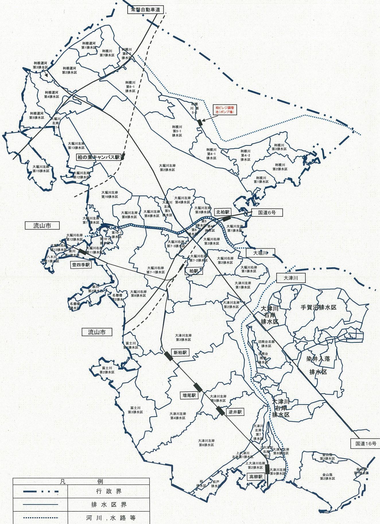
図1-2 雨水計画図
