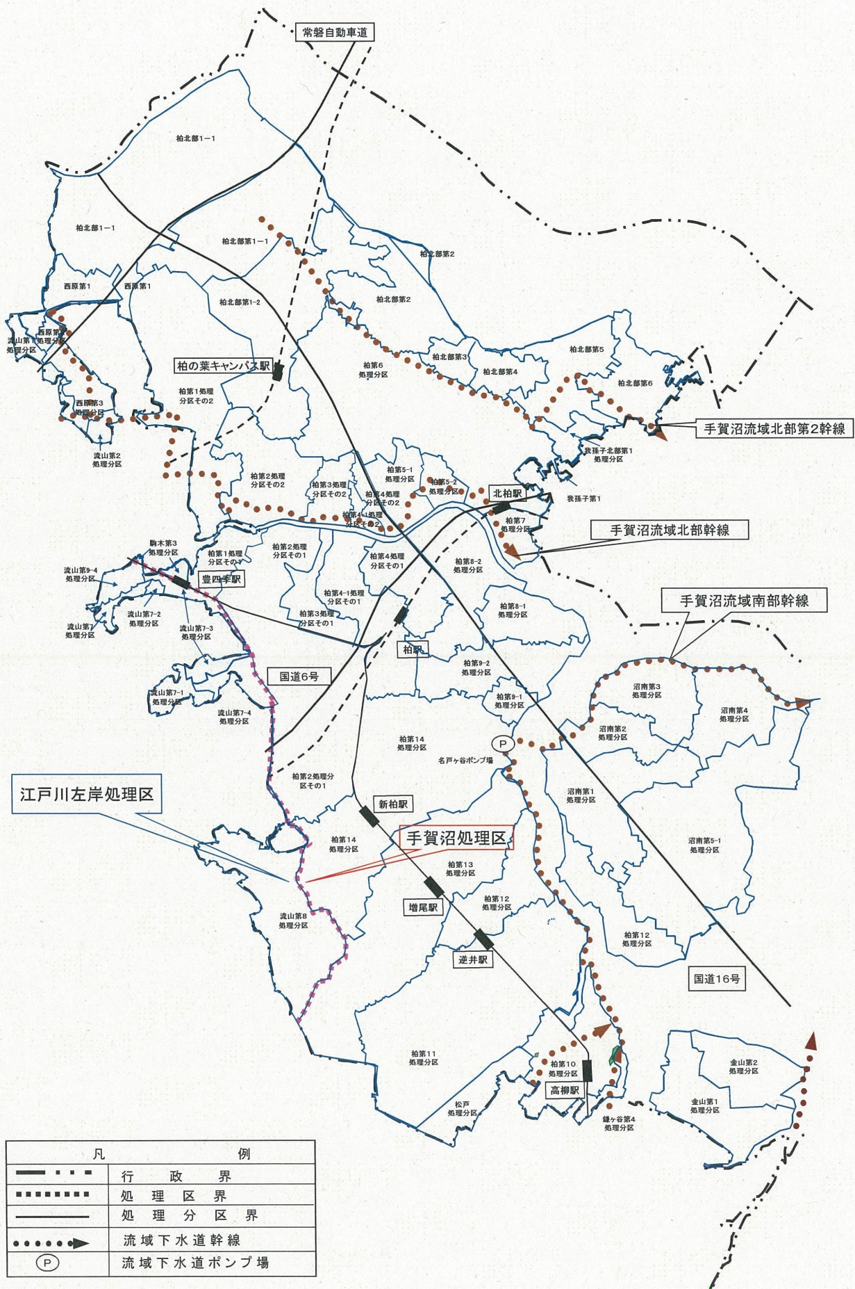
図1-1 汚水計画図
