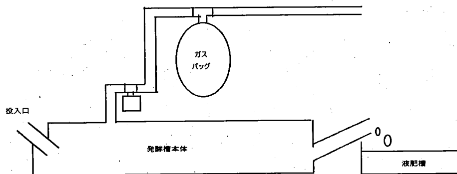
バイオガス基構造 簡素図
