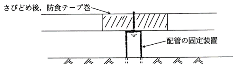
例図2 配管の固定装置の部分
