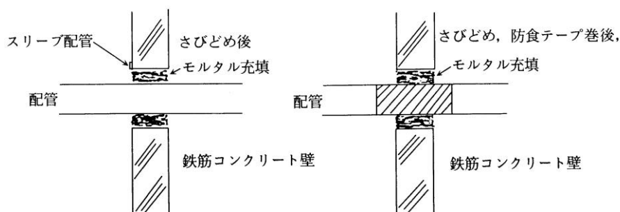
例図2 配管の固定装置の部分
