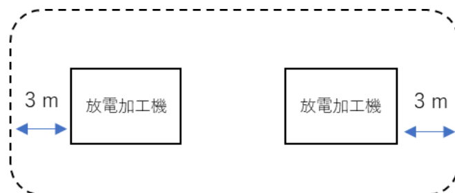
複数の機器を設ける場合の空地の例
