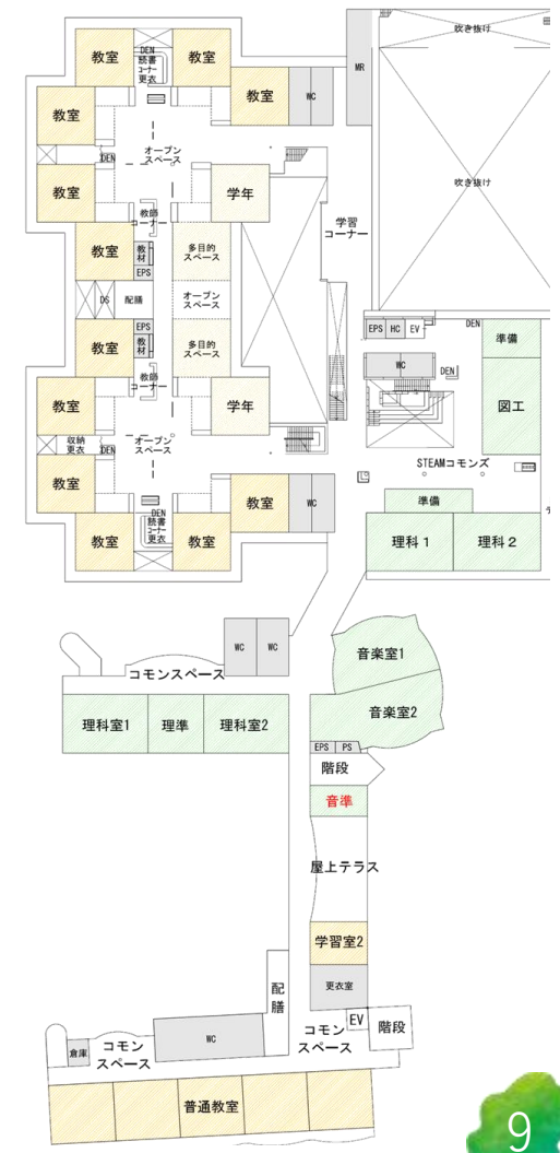
4F平面図
