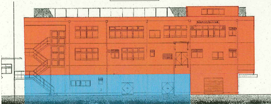
旧庁舎立面図
