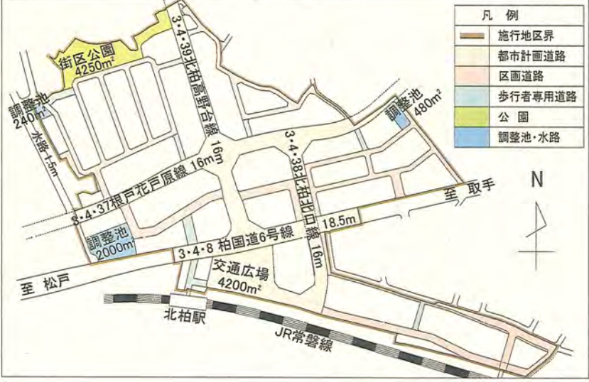
北柏駅北口土地区画整理事業計画図
