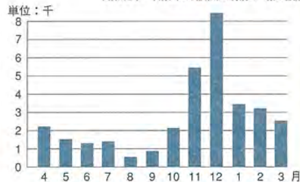
年末は交通量が増えるうえ、上空の暖気と地表の冷気の境目に、地表の汚れた空気を閉じ込める層(逆転層)ができやすく、1年で最も大気が汚れます
