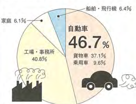
■図2 NOx排出量の発生源別内訳[7都県市]
