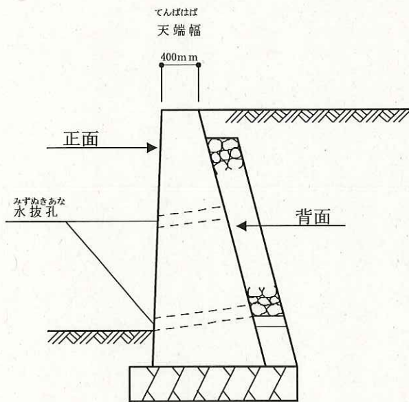
じゆうりよくしき 重力式コンクリート擁壁の例
