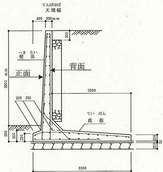
てつきん 鉄筋コンクリートL型擁壁の例
